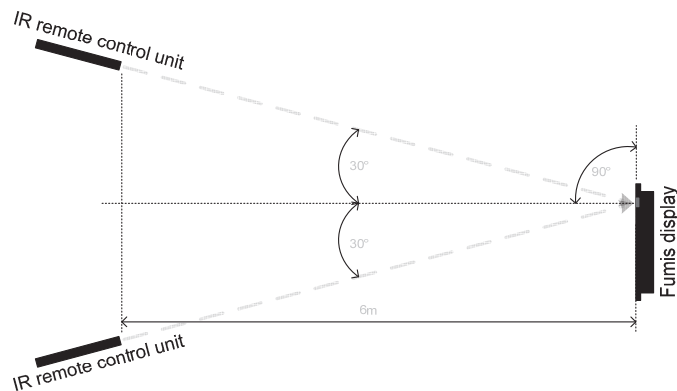
Abbildung 2: IR-Fernbedienung (Betriebswinkel)
